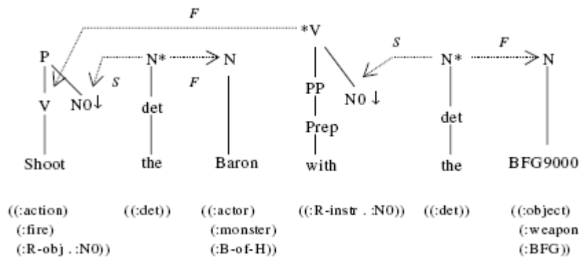
Gambar 4. Integrasi Sintaks-semantik
